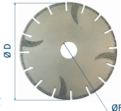
A settori con razze Discontinuous rim with pads
